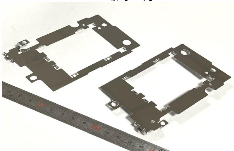
タッチプレート【プリンター】
